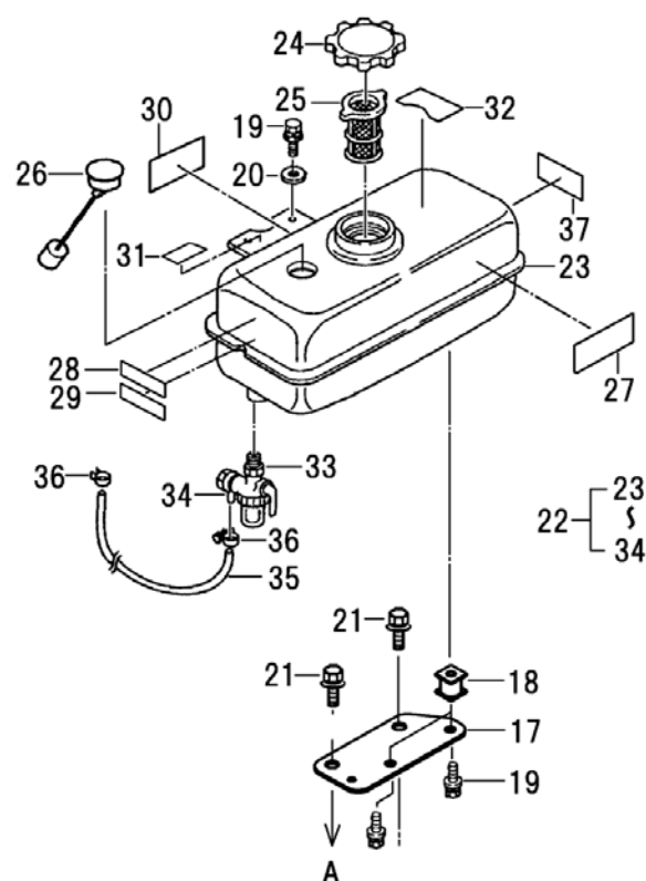
FIG.104 ファンカバー, 燃料タンク (FUN COVER,FUEL TANK)
