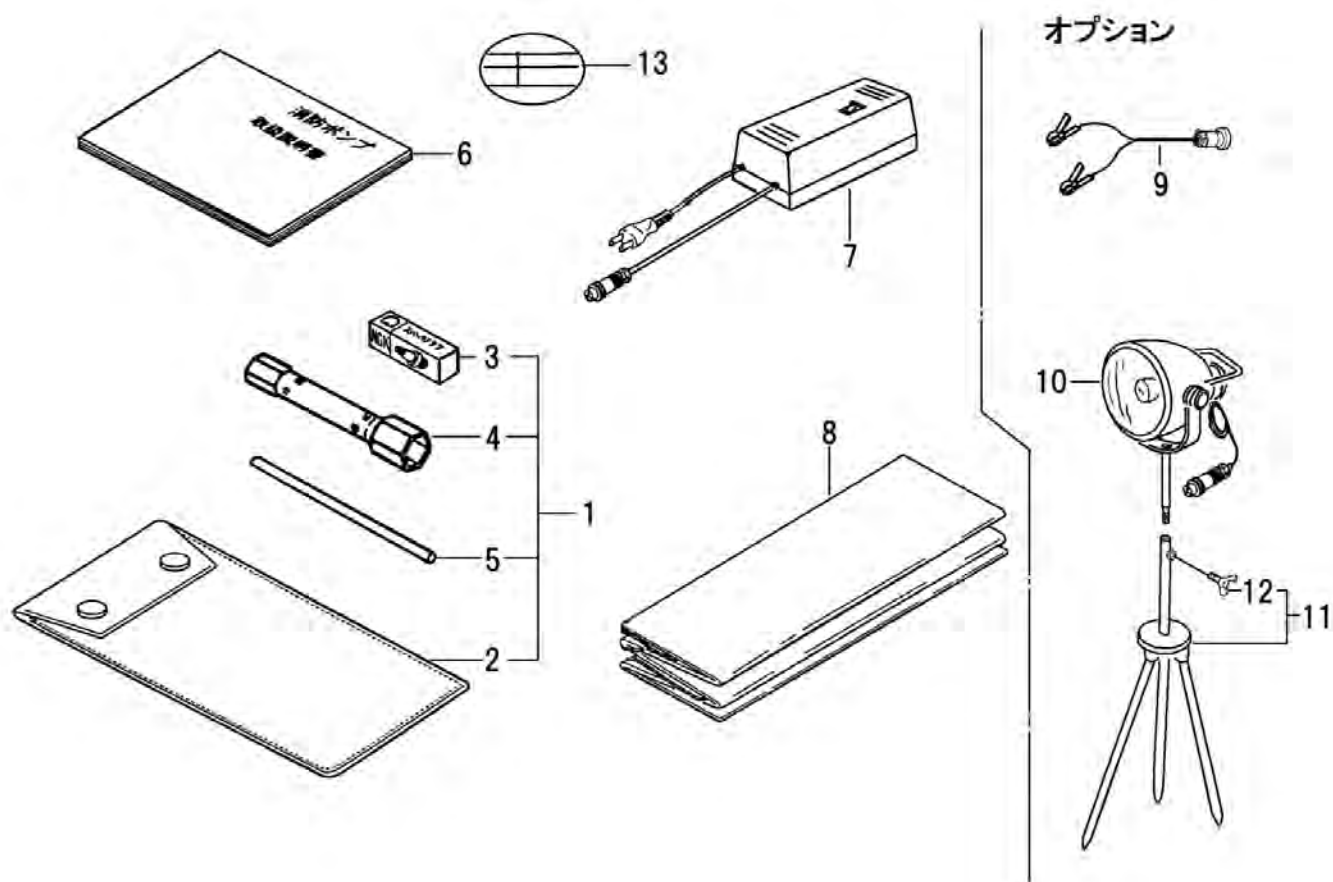
FIG.115 ツール,オプションパーツ (TOOLS、OPTIONS PARTS)
