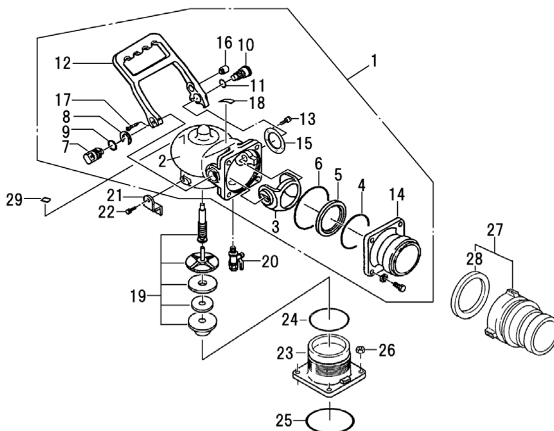
FIG.109 デリバリバルブ (DELIVERY VALVE)
