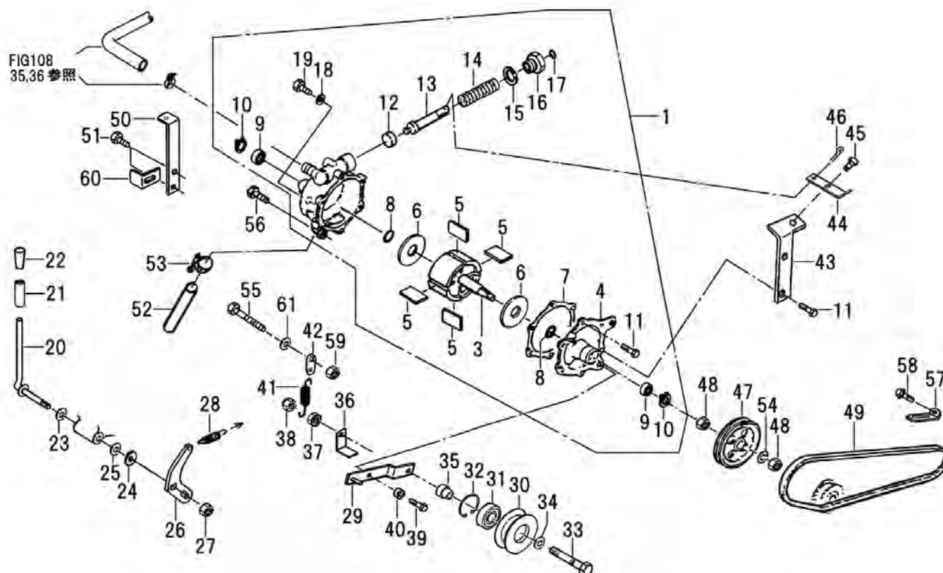
FIG.110 バキュームポンプ (VACUUM PUMP)
