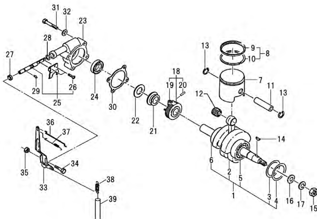
FIG.102 クランクシャフト, ガバナ (CRANK SHAFT, GOVERNOR)
