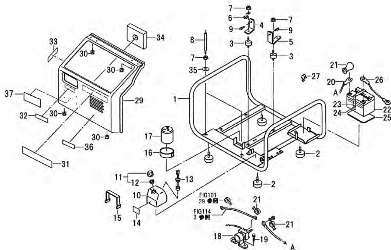
FIG.111 ベッド, カバー (BED,COVER)
